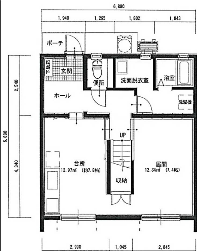
1階平面図
