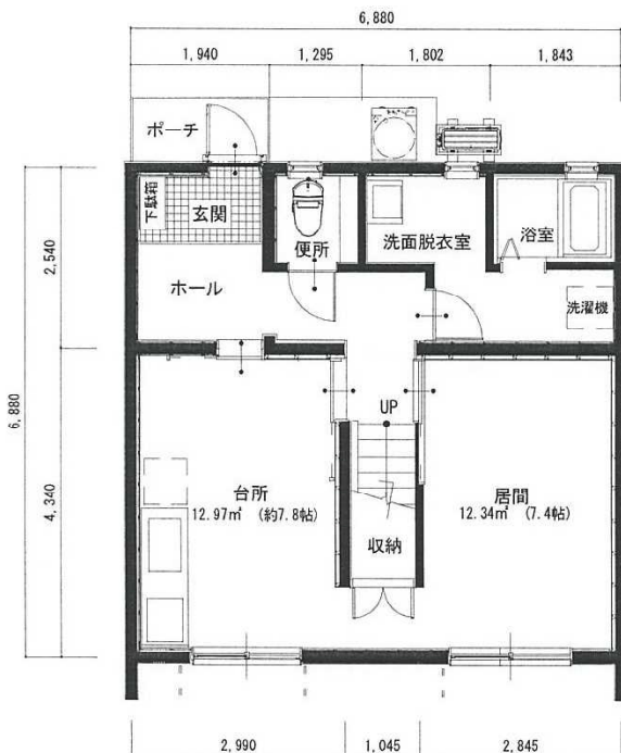
1階平面図
