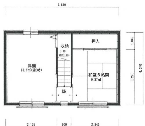
2階平面図
